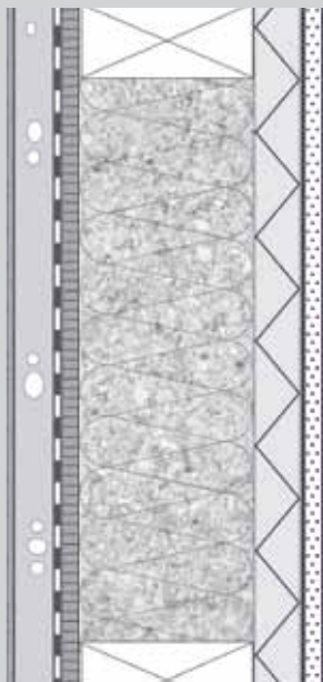
Vakolt homlokzatú favázás fal
